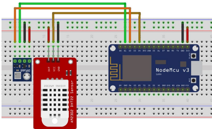
სურ.137. სენსორების დაერთება NodeMCU-ზე
