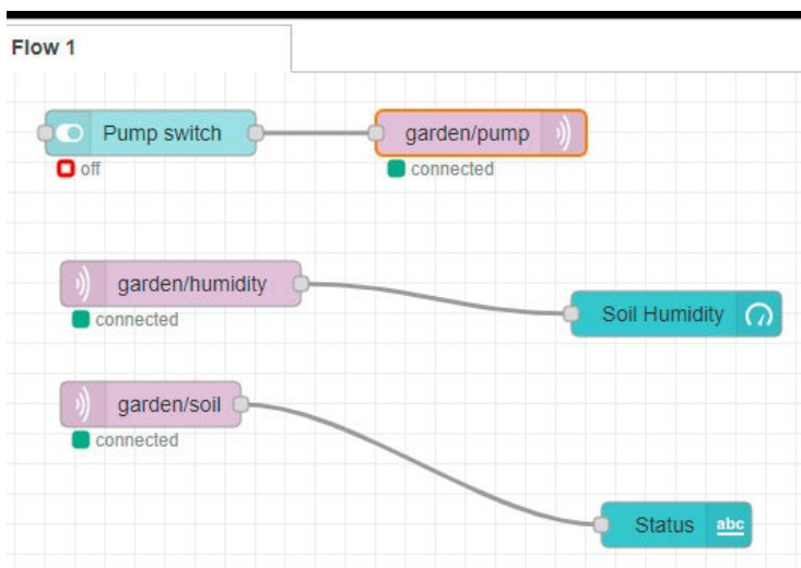
სურ. 110. კვანძების დაკავშირება
