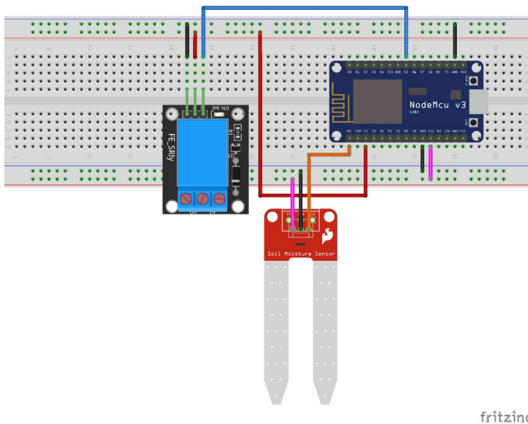
სურ.109 . მარტივი სარწყავი სისტემის სქემა
