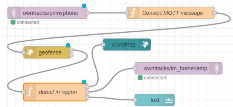
სურ. 143 . კვანძების დაკავშირება
