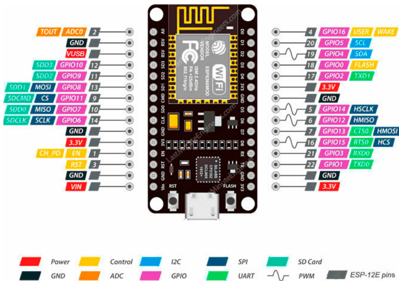
სურ. 26. NodeMCU-ს საკონტაქტო გამომყვანების განლაგება
